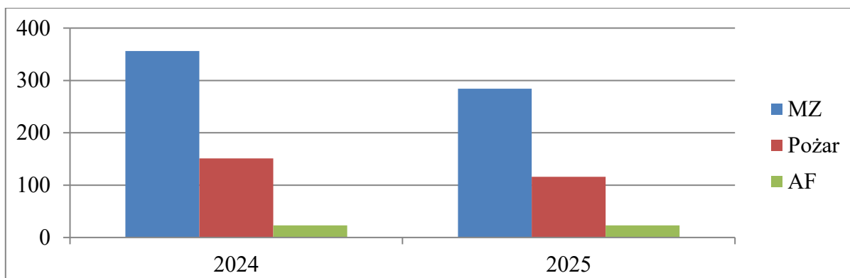
Struktura zdarzeń
